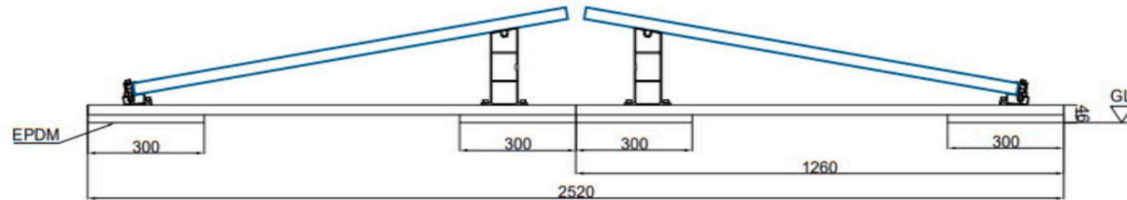
Seitenansicht (Ost/West Ausrichtung)
